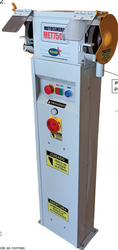
Exposição máxima do rebolo Norma NBR 15230
